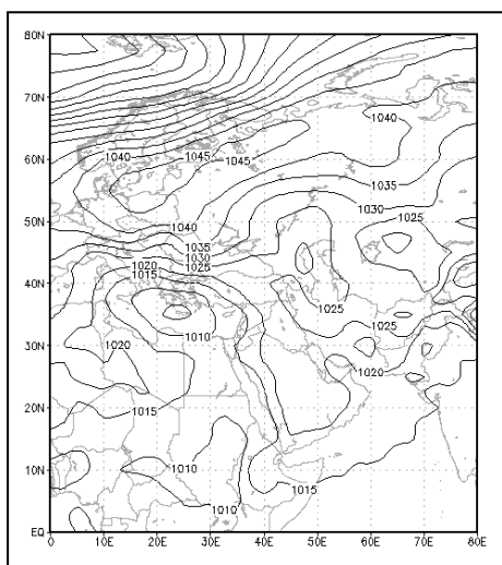
شکل ۴: الگوی گردشگری فشار سطح دریا در روز ۲۳ ژانویه سال ۲۰۰۶
