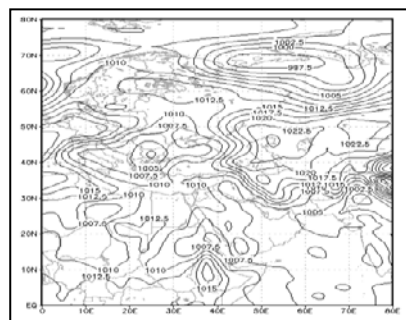
شکل ۱۰ الگوی گردشی فشار سطح دریا در روز ۱۸ مه سال
