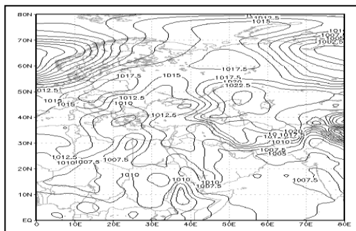
شکل ۱۱: الگوی گردشی فشار سطح دریا در روز ۱۹ مه سال ۲۰۰۷
