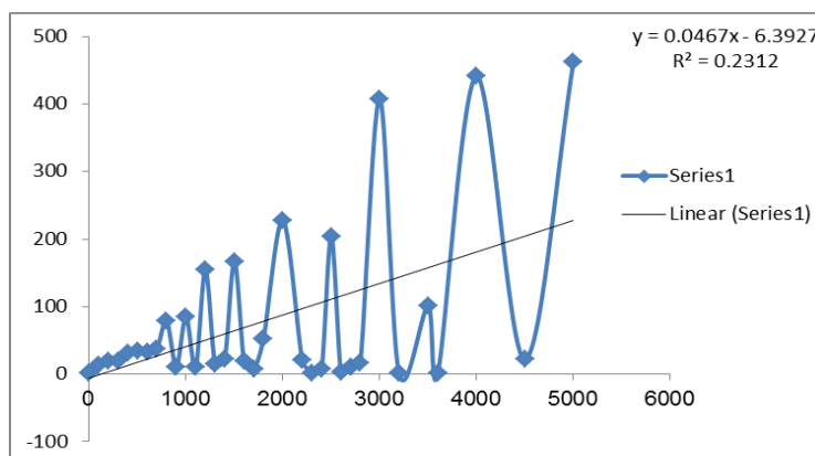
شکل ۱: نمودار بسامد اختلالات پروازی فرودگاه بین‌المللی اهواز پدیده‌ی گرد و خاک (کد ۰۶) در ایستگاه هم‌دید اهواز
