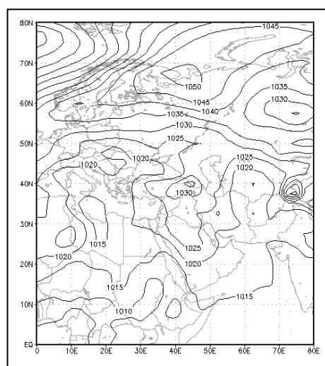
شکل ۳: الگوی گردشگری فشار سطح دریا در روز ۲۲ ژانویه سال ۲۰۰۶
