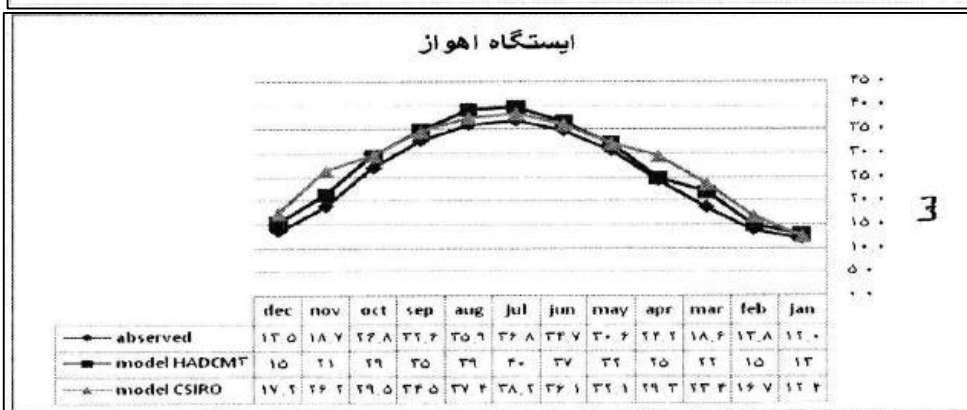
شکل ۳- رژیم میانگین دمای ماهانه براساس مدل HadCM3 و CSIRO تحت سناریوی A2 و B1
