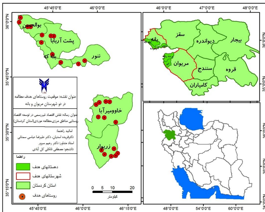
شکل ۲. موقعیت روستاهای هدف مطالعه در دو شهرستان مریوان و بانه نسبت به کشور منبع: (سازمان جغرافیایی نیروهای مسلح)
