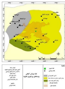
شکل ۶. پوشش گیاهی
