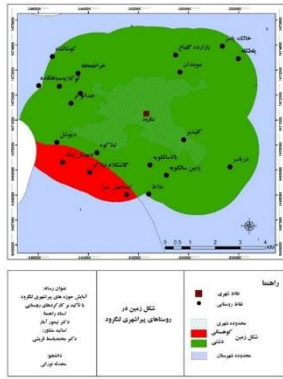
شکل ۴. شکل زمین
