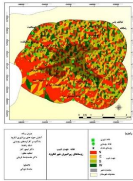
شکل ۳. جهت شیب
