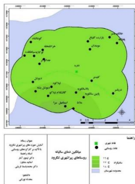
شکل ۸. میانگین دما
