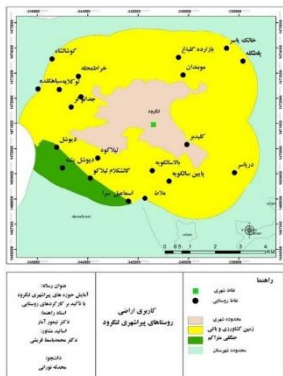
شکل ۷. کاربری اراضی
