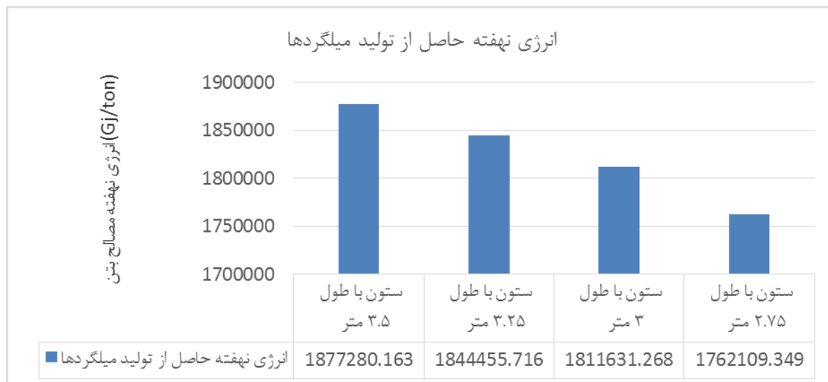
نمودار ۵. مقایسه مقادیر انرژی نهفته حاصل از تولید میلگرد
