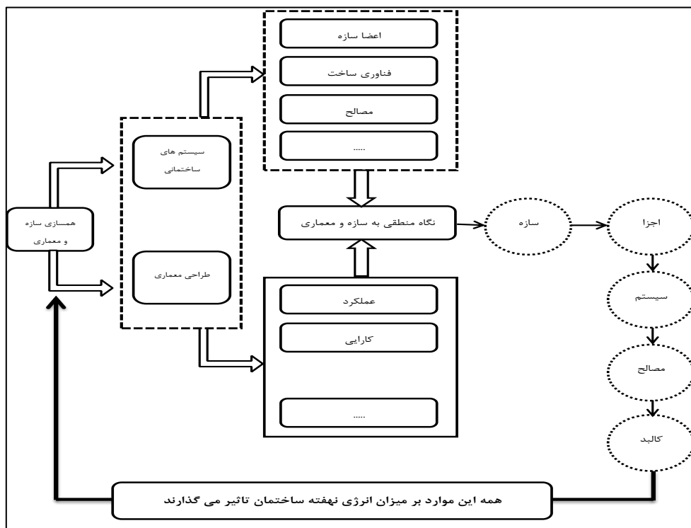
نمودار ۲: همسازی سازه و معماری در انرژی نهفته
