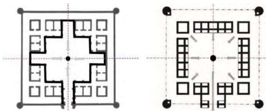
تصویر ۶. مرکزیت، محور بندی و تقارن در کاروانسراهای دوره صفویه
