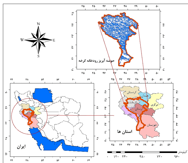
شکل ۳- نقشه موقعیت جغرافیایی حوضه آبریز رودخانه کرخه
