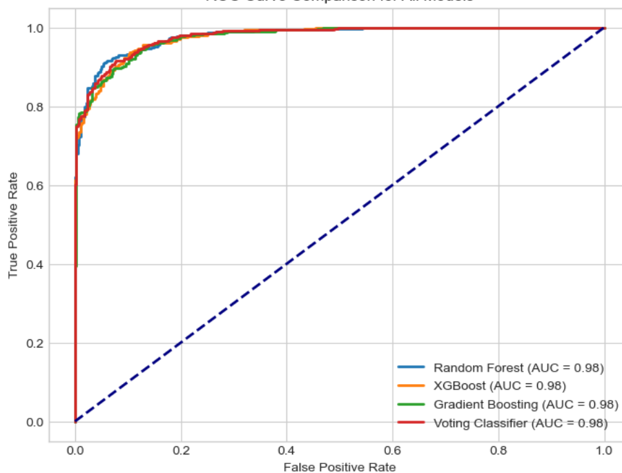
شکل ۵. مقایسه منحنی‌های ROC مدل‌های مختلف با AUC برابر ۰/۹۸ برای ارزیابی توانایی تفکیک نمونه‌های "پایدار" و "ناپایدار" توسط مدل‌ها
