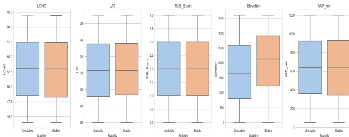
شکل ۴. مقایسه توزیع ویژگی‌های مختلف در دو کلاس "پایدار" و "ناپایدار" با استفاده از نمودارهای جعبه‌ای، که نشان‌دهنده تفاوت‌های پراکندگی و میانه در هر ویژگی است
