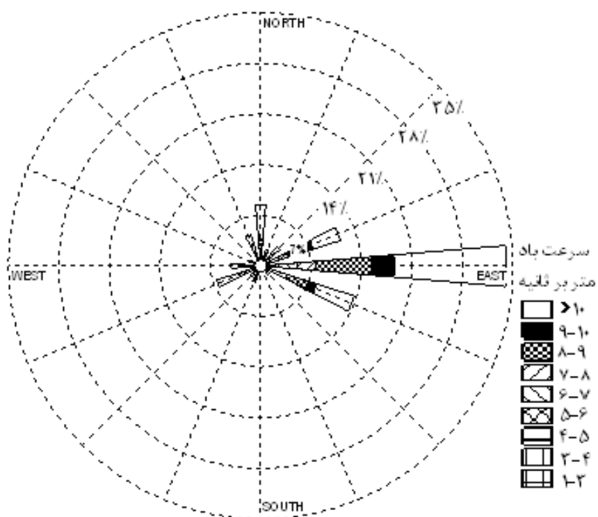
شکل ۲- گلباد سالیانه ایستگاه سینوپتیک سبزوار در دوره آماری ۱۳۶۷ تا ۱۳۸۷
