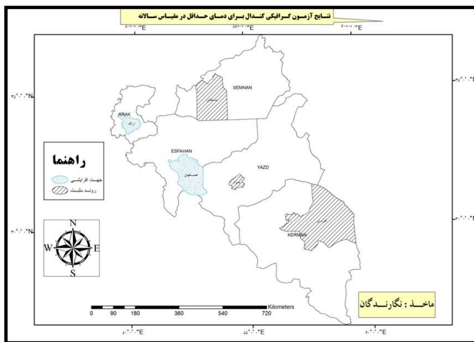
شکل ۲: نتایج آزمون گرافیکی کندال برای دمای حداقل در مقیاس سالانه
