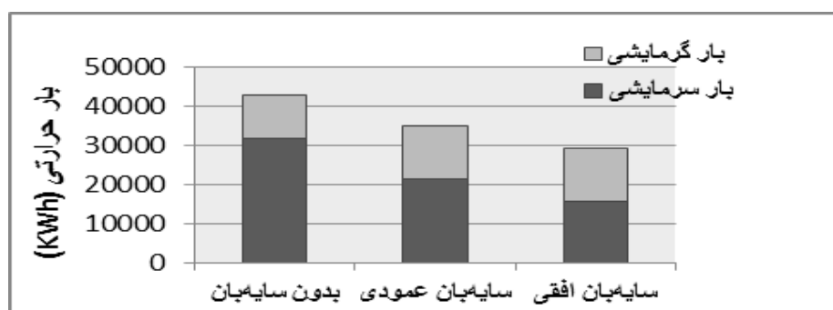
نمودار ۴- میزان بار حرارتی در سه حالت بدون سایه‌بان و سایه‌بان افقی و عمودی در ماه‌های جولای و دسامبر با استفاده از Energy Plus
