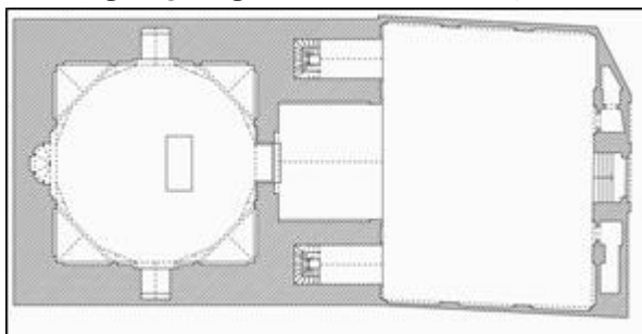
نقشه ۸: پلان مدرسه سید رکن‌الدین (آرشیو اداره کل میراث فرهنگی، صنایع دستی و گردشگری استان یزد)
