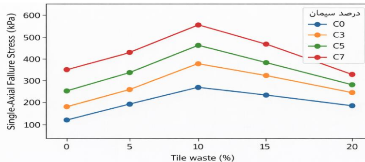
شکل ۵. تغییرات تنش گسیختگی تک‌محوری ( q_{II} ) خاک مارن بر حسب درصد پودر ضایعات کاشی در سطوح مختلف سیمان (عمل‌آوری ۲۸ روزه)
