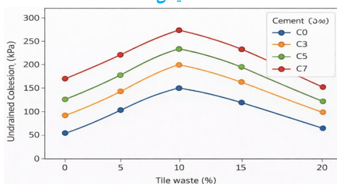
شکل ۸. تغییرات چسبندگی زهکشی‌نشده ( C_{II} ) خاک مارن تثبیت‌شده بر حسب درصد پودر ضایعات کاشی در سطوح مختلف سیمان (عمل‌آوری ۲۸ روزه)
