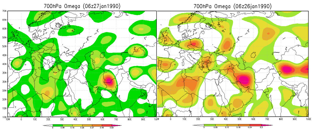
شکل ۳: نقشه امگا تراز ۷۰۰ hpa در ساعت 00,06 UTC در روز ۲۶ و ۲۷ ژانویه ۱۹۹۰
