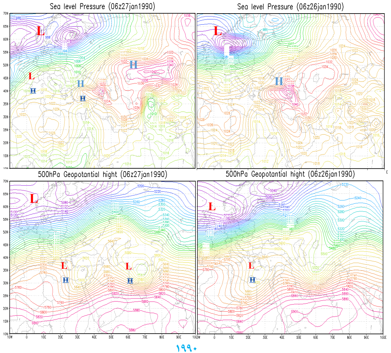
شکل ۲: توزیع فشار تراز دریا و ۵۰۰ هکتوپاسکال در ساعت 00,06 UTC در روزهای ۲۶ و ۲۷ ژانویه
