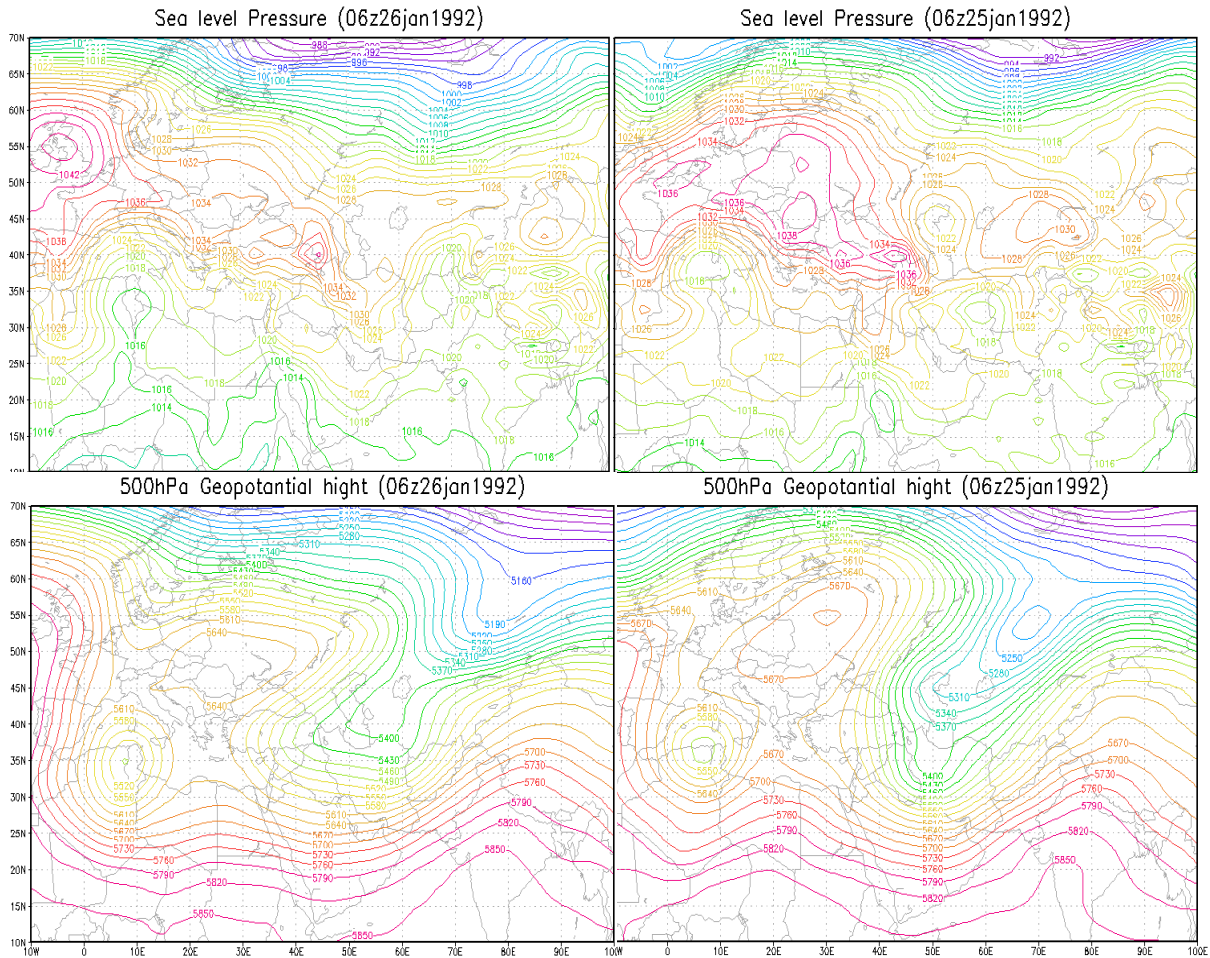
شکل ۸: توزیع الگوی فشار تراز دریا و hpa 500 در ساعت 00,06 UTC در روزهای ۲۵ تا ۲۶ ژانویه ۱۹۹۲
