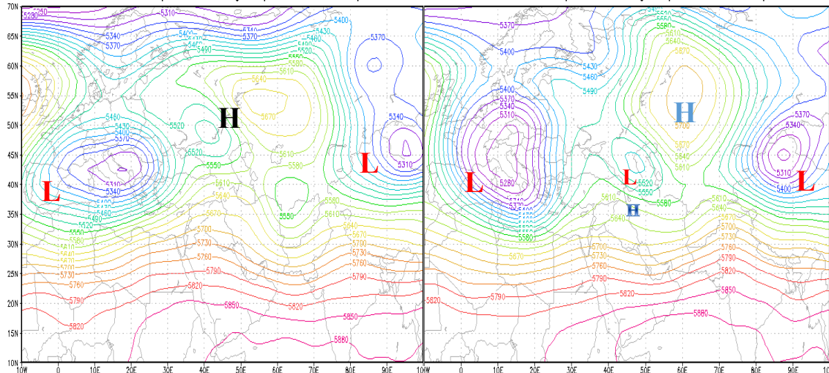
شکل ۶: توزیع الگوی فشار تراز دریا و ۵۰۰ hpa در ساعت 00,06 UTC در روزهای ۲۶ و ۲۷ فوریه
