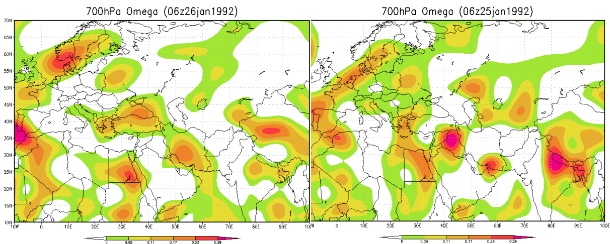
شکل ۹: نقشه امگا تراز hpa 700 در ساعت 00,06 UTC در روزهای ۲۵ تا ۲۶ ژانویه ۱۹۹۲
