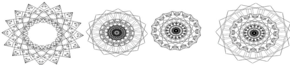
شکل ۷: الگوهای هندسی
