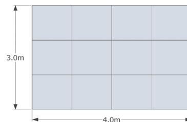
شکل ۲: مستطیل ۳ در ۴
